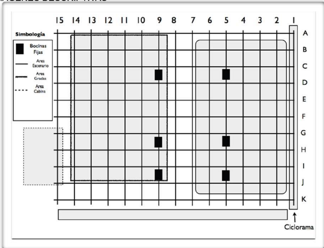
FIG 1. Configuración convencional y más usada del Foro Experimental.
